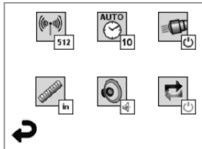
Εικόνα 7 – Μενού εργαλείων
